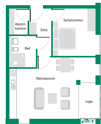
Musterbeispiel einer Zweizimmer-Wohnung im Betreuten Wohnen.
