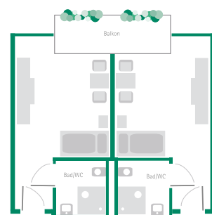
Der Grundriss zeigt das Beispiel eines 1-Bett-Pflegezimmers mit einer Größe von 21 m 2 .
