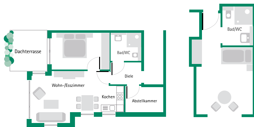
Der Grundriss zeigt die Wohnbeispiele im Betreuten Wohnen
