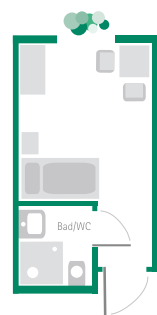
Der Grundriss zeigt das Beispiel eines 1-Bett-Pflegezimmers mit einer Größe von 22 m 2 .
