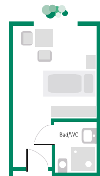
Musterbeispiel eines Einzelzimmers der ambulanten Wohngemeinschaft
